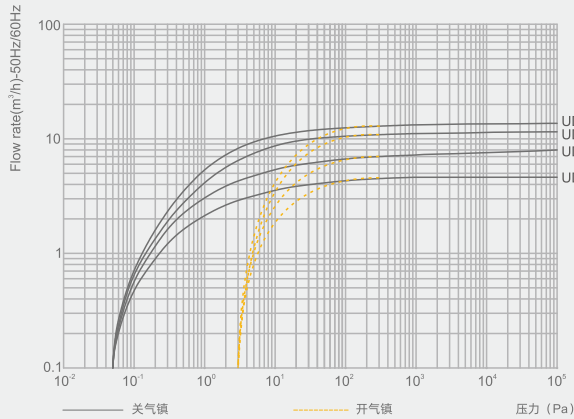
抽气速率曲线图
