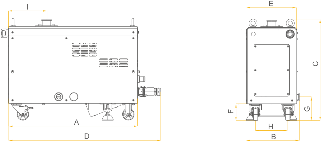
图1 VSU102/104/106 产品尺寸
