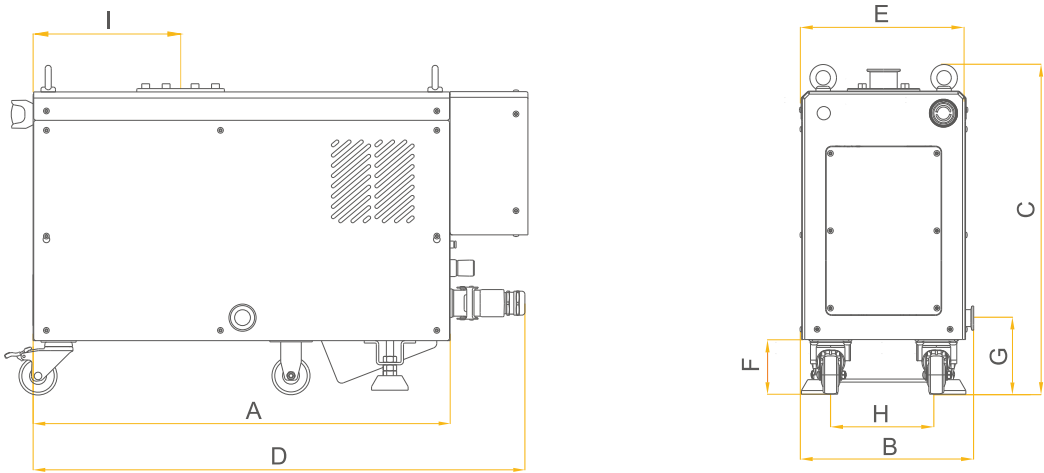
图2 VSU206 产品尺寸
