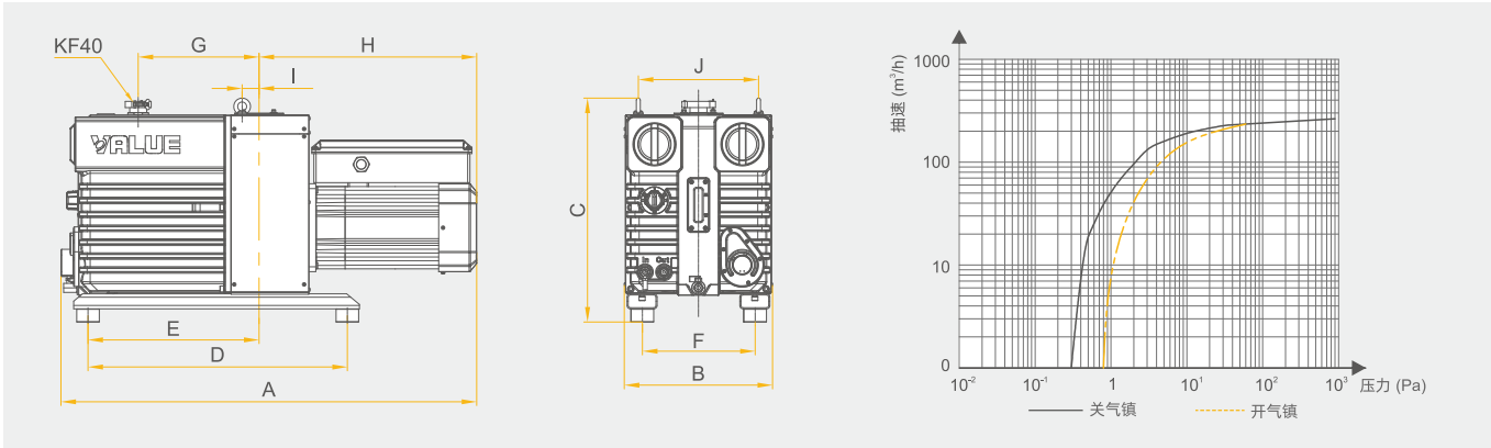
尺寸(单位: mm)
